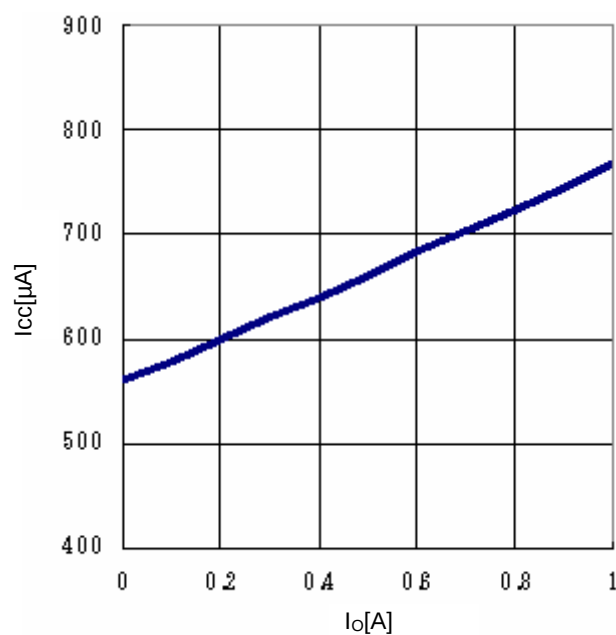
Fig.20 I_o - I_{cc}
