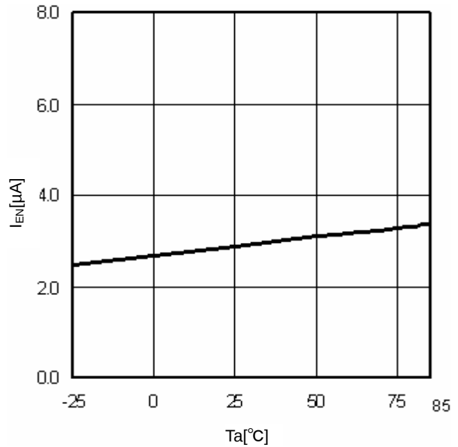
Fig.12 T_a - I_{EN}
