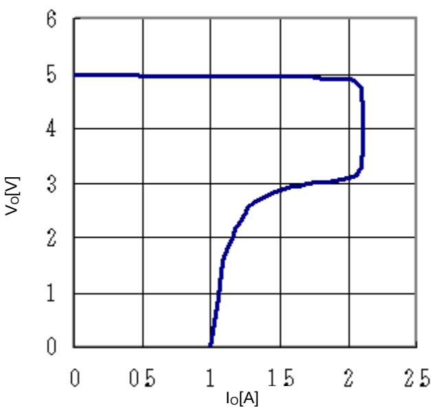
Fig.17 OCP
