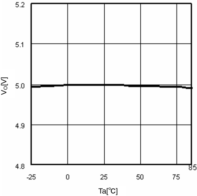
Fig.9 T_a-V_O ( I_o=0mA )
