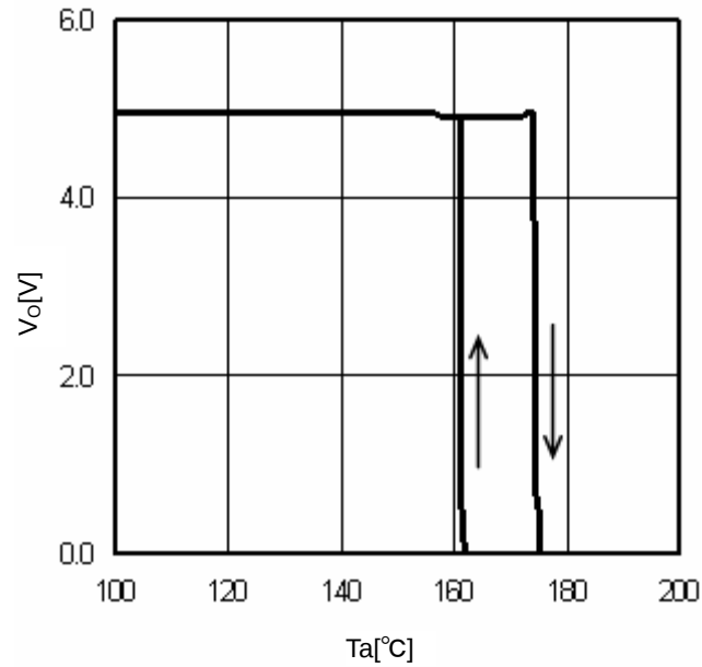
Fig.16 TSD ( I_O=0mA )
