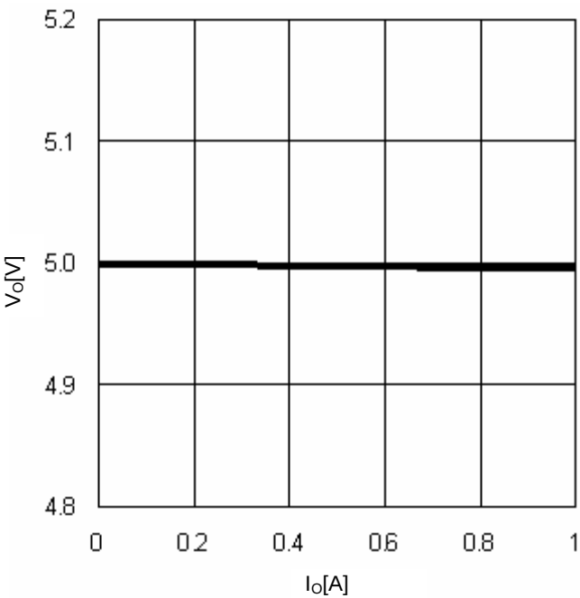
Fig.13 I_O - V_O
