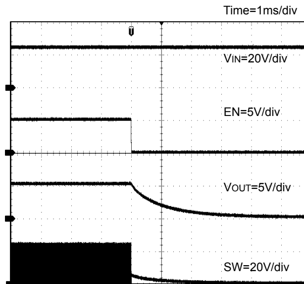
Figure 22. Power Down (EN = 5V→0V) (VOUT = 5.0V)
