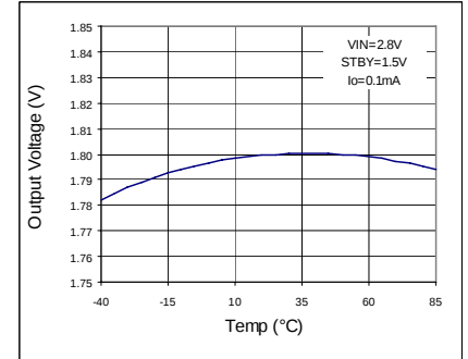
Fig 11. VOUT - Temp
