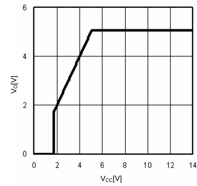
Fig.15 V CC -V O (I O =0mA)
