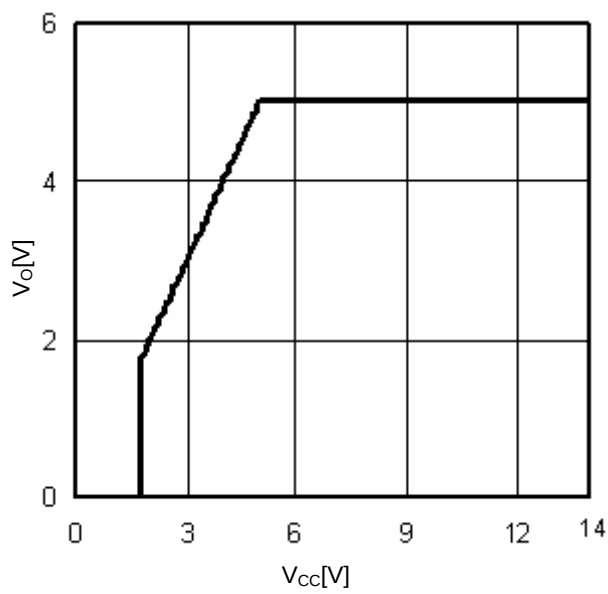
Fig.15 V_{CC}-V_O ( I_O=0mA )
