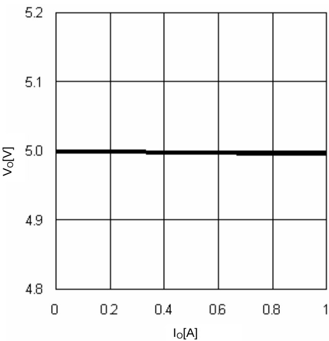
Fig.13 I_O - V_O
