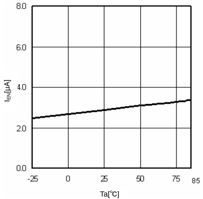
Fig.12 T_a - I_{EN}
