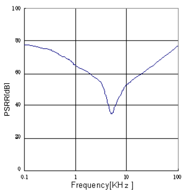
Figure 21. PSRR (Io=0mA)
