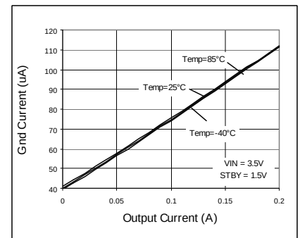
Fig. 100 IOU - IGND
